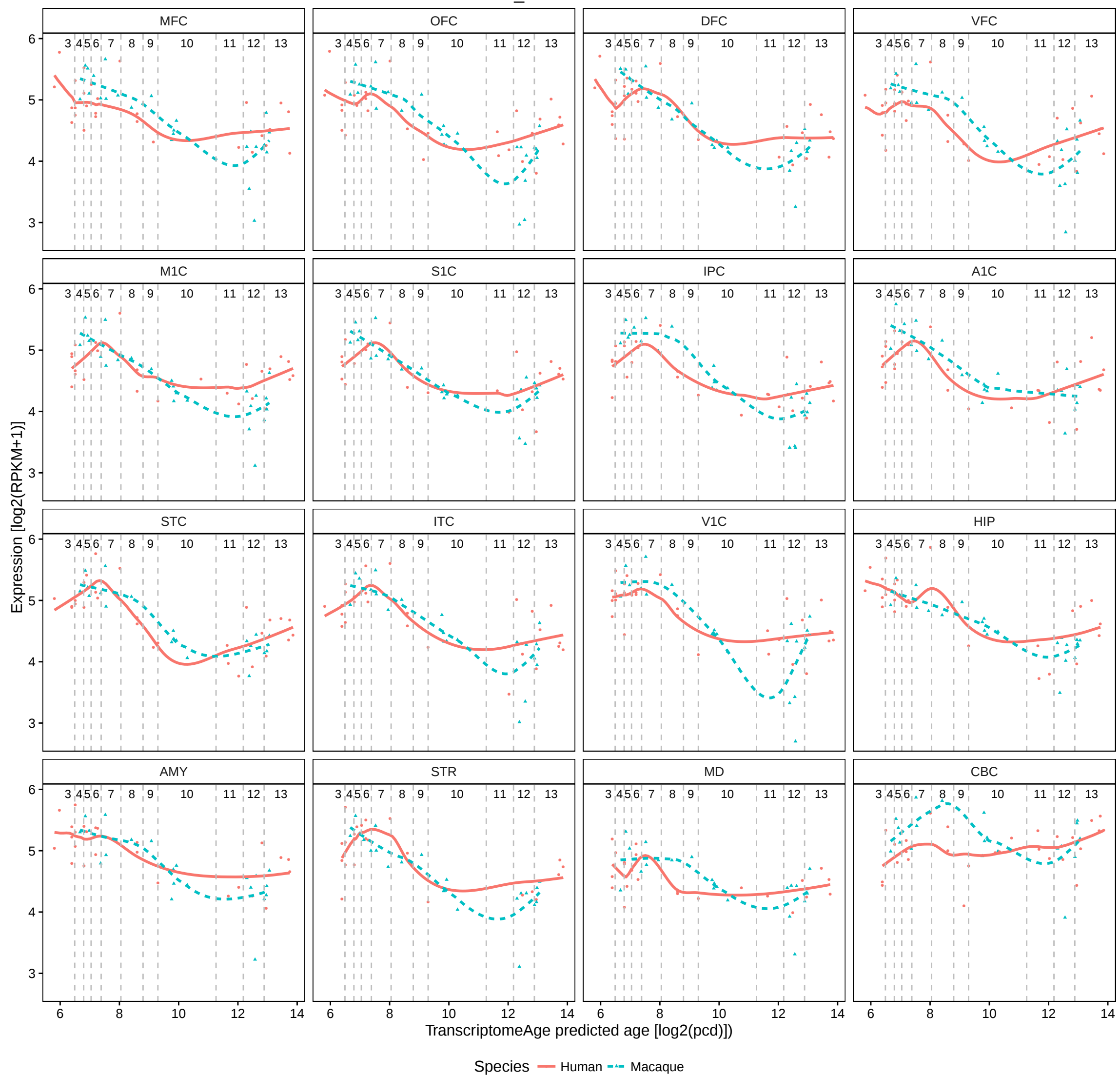
TAB1_ENSG00000100324
